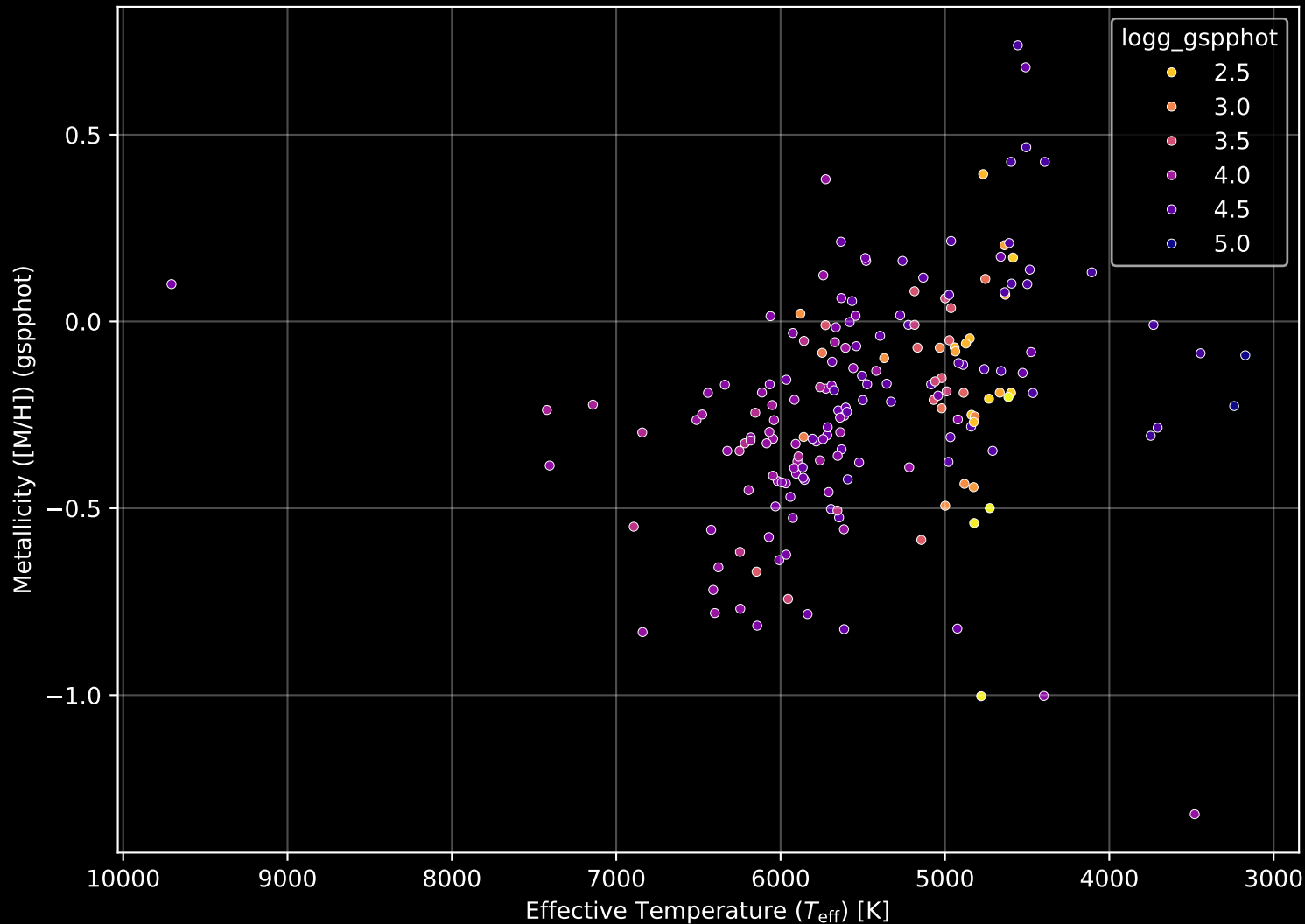
APOGEE DR17 Field: [177+51_MGA] Stellar Population Parameters (n= 189)
